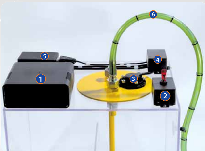
Dieseltankmodell
