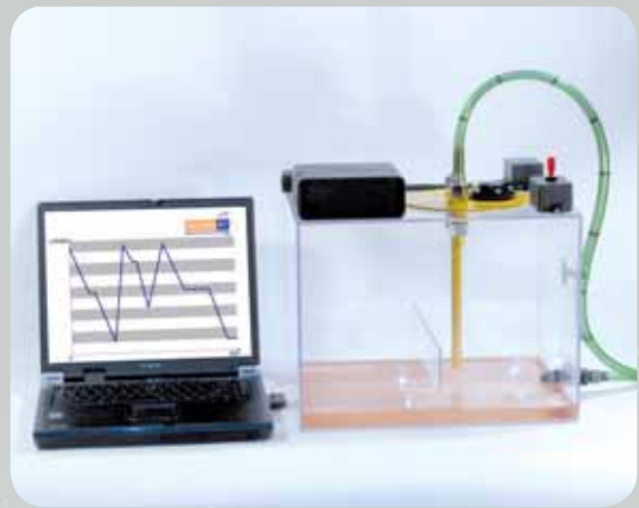
Dieseltankmodell angeschlossen an einen Computer
